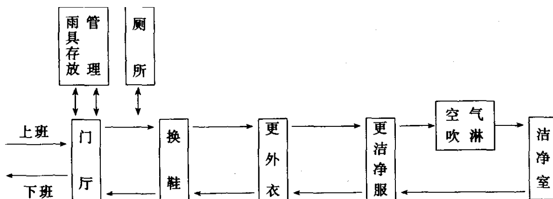
图 4.3.4 人员净化程序
